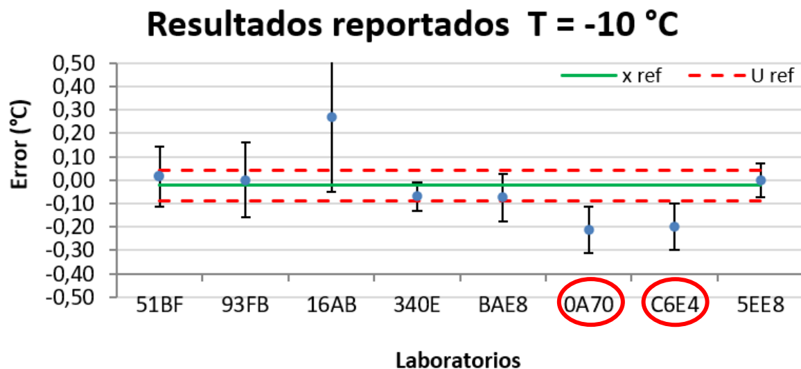
Figura 8. Resultados para T = -10\text{ }^{\circ}\text{C} : Laboratorio de temperatura del IBMETRO, 2023
