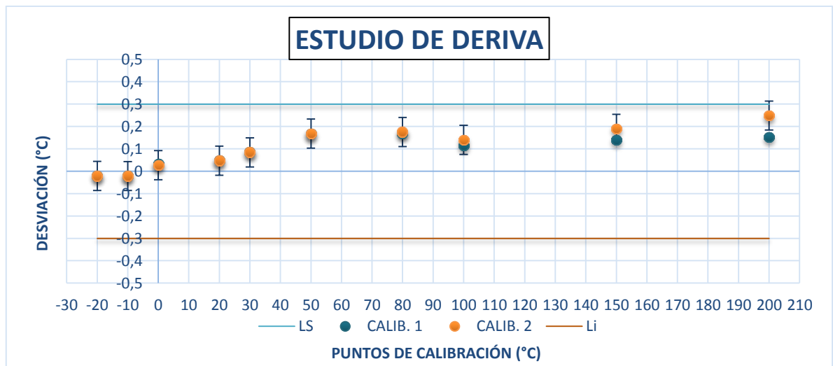
Figura 4. Resultados del estudio de deriva realizado al ítem de ensayo IBM011040209 (Barras de error) e intervalo de cobertura al 95 % de confianza para el valor asignado en cada punto de calibración evaluado.
