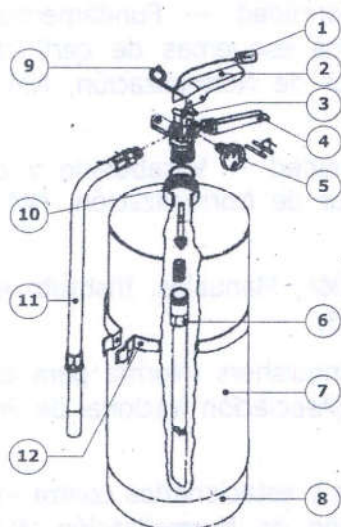
Figura 1. Partes de un extintor de polvo químico seco presurizado.
