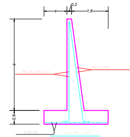
MURO SECTOR TANQUE DE AGUA
