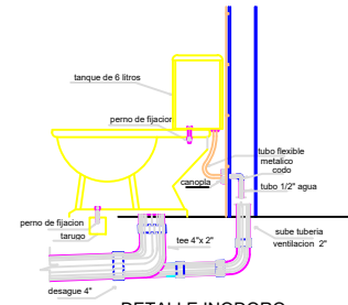
DETALLE INODORO
