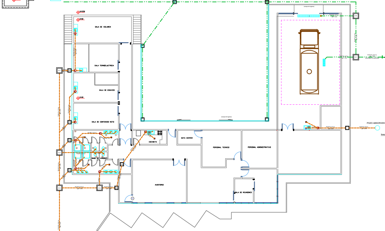
PLANO EN PLANTA SISTEMA SANITARIO
