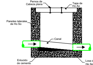
DETALLES CÁMARA DE INSPECCIÓN
