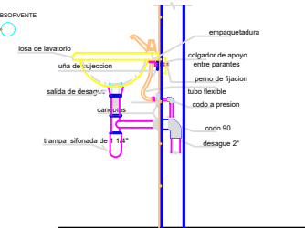
DETALLE LAVAMANOS
